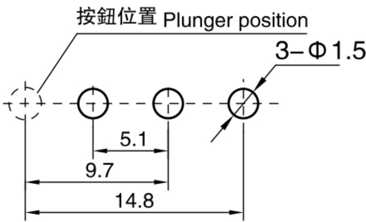
PCB端子 PCB terminal
